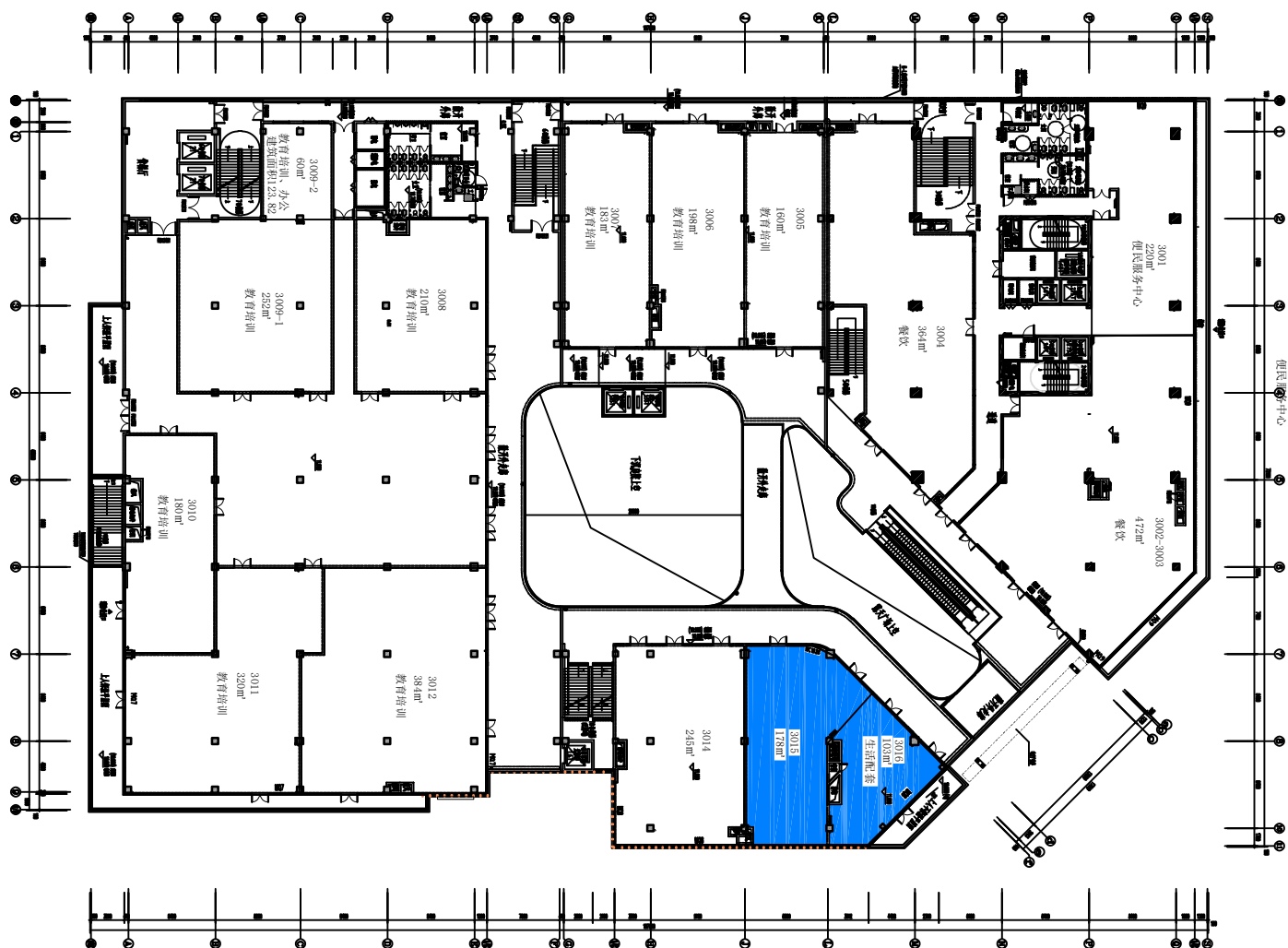
三层平面图
